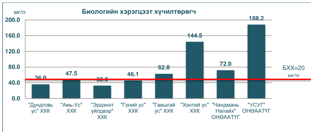
Зураг 5. Цэвэрлэх байгууламжаас хүрээлэн буй орчинд нийлүүлж буй хаягдал усан дах БХХ
